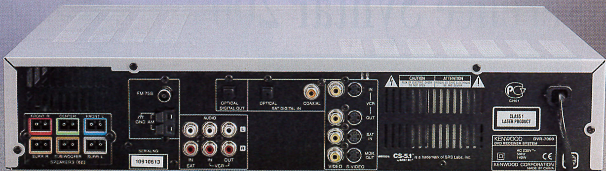
Il retro mostra una completa dotazione di connessioni.
